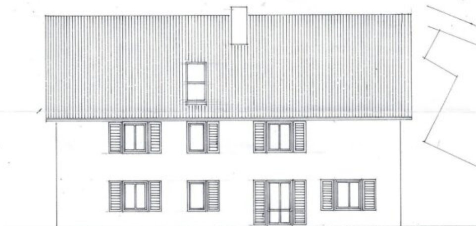
ANSICHT OST
