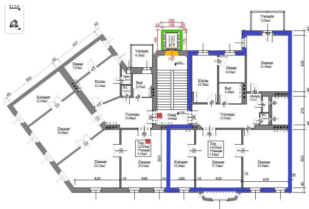
Grundriss 2. Stock 1:100
