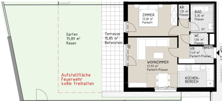
ÜBERSICHTSPLAN-EG
