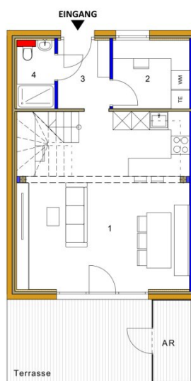
Erdgeschoss M1:75
