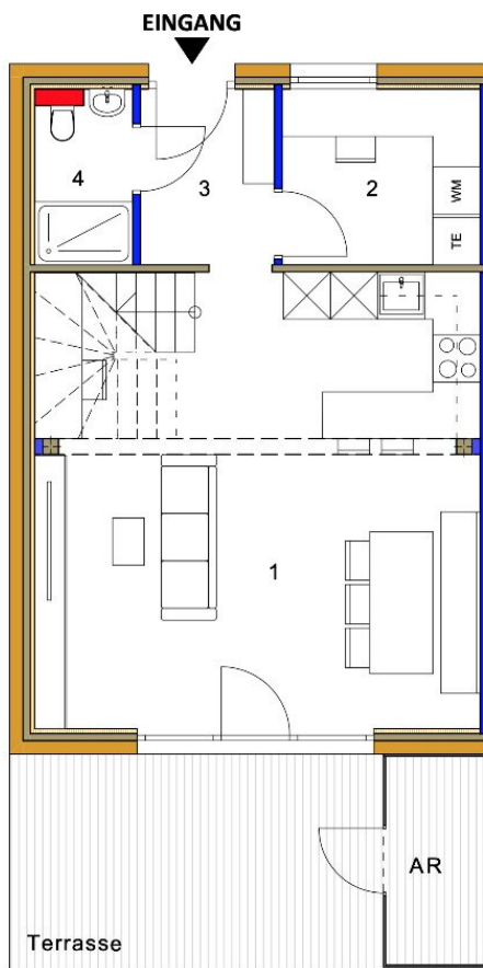
Erdgeschoss M1:75
