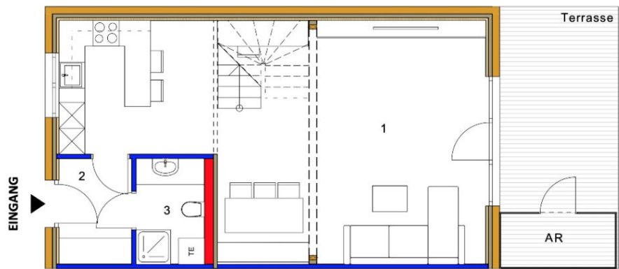
Erdgeschoss M1:75
