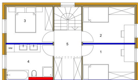
Obergeschoss M1:75
