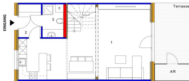
Erdgeschoss M1:75
