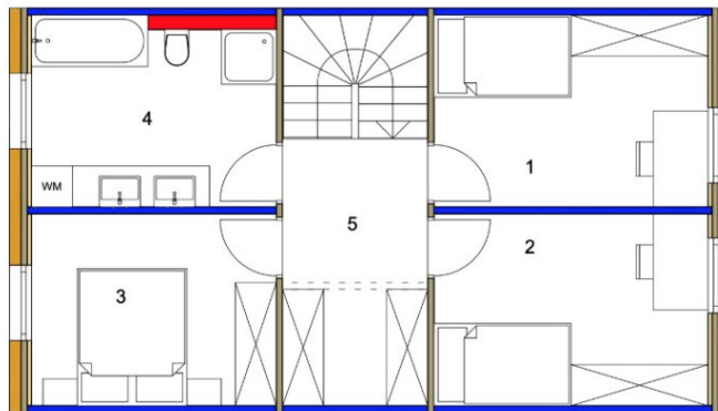
Obergeschoss M1:75
