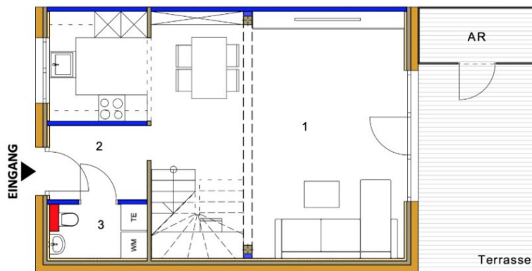
Erdgeschoss M1:75
