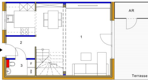
Erdgeschoss M1:75
