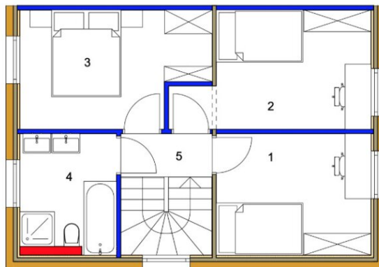
Obergeschoss M1:75
