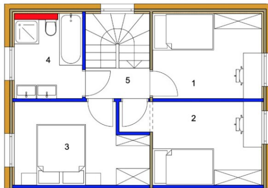
Obergeschoss M1:75
