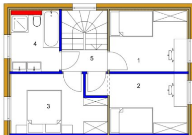
Obergeschoss M1:75
