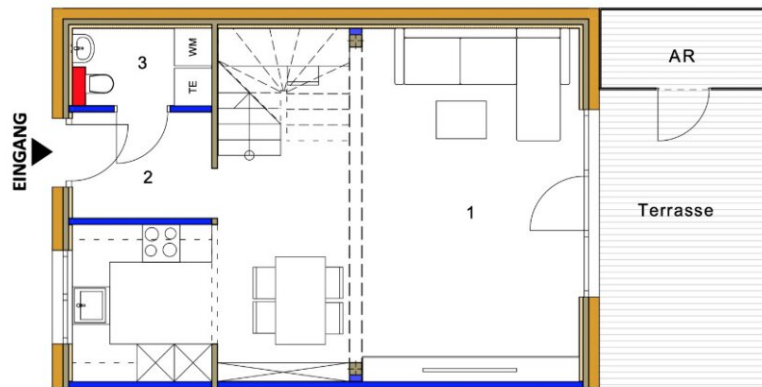
Erdgeschoss M1:75
