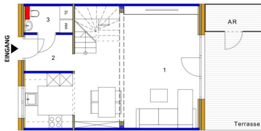
Erdgeschoss M1:75
