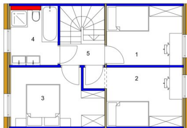
Obergeschoss M1:75
