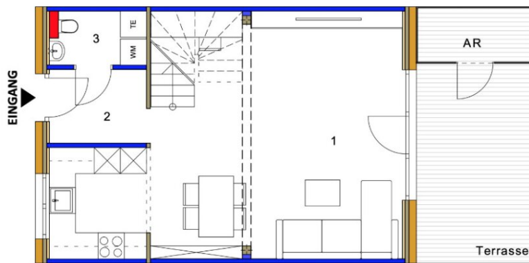
Erdgeschoss M1:75
