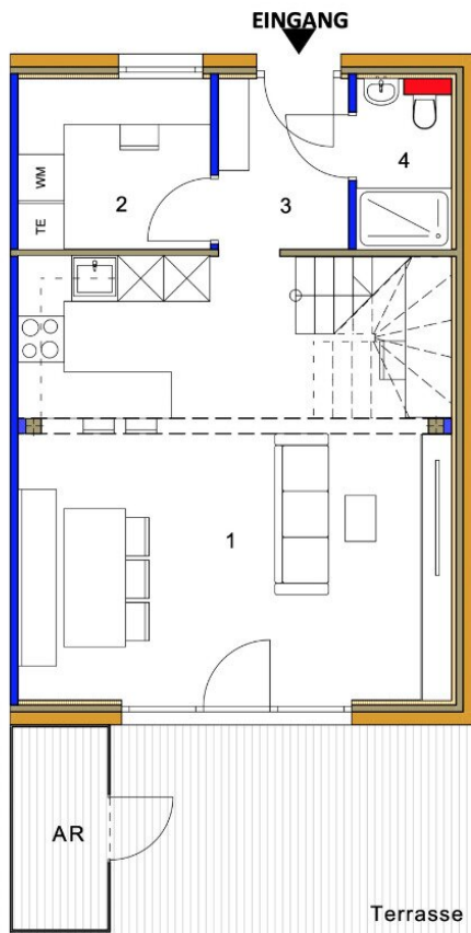
Erdgeschoss M1:75
