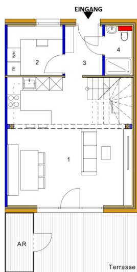
Erdgeschoss M1:75
