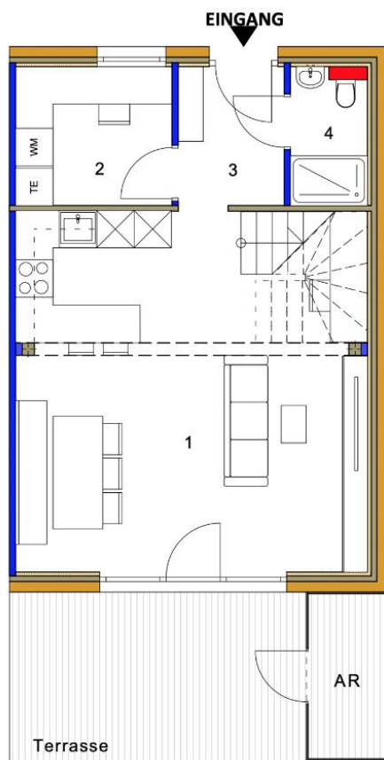
Erdgeschoss M1:75
