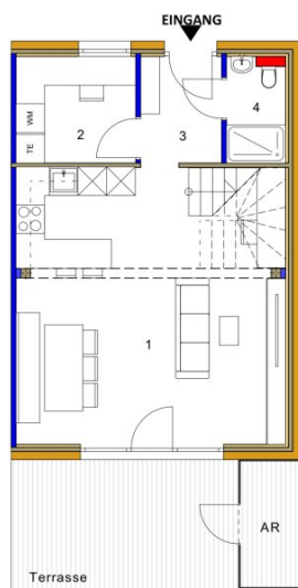
Erdgeschoss M1:75
