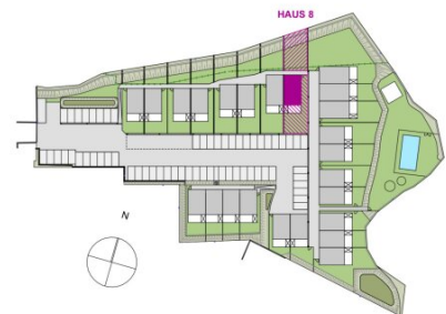
Übersicht | Lage
