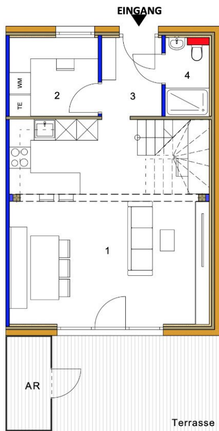
Erdgeschoss M1:75
