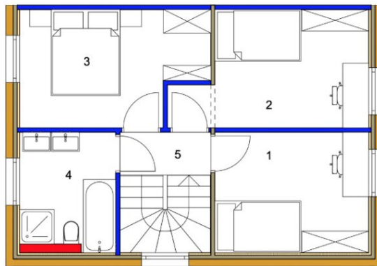
Obergeschoss M1:75
