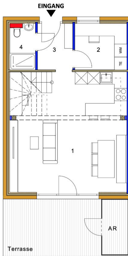
Erdgeschoss M1:75
