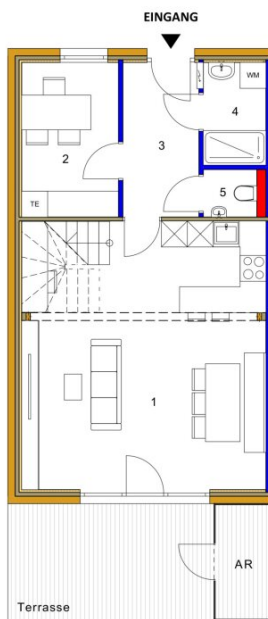
Erdgeschoss M1:75
