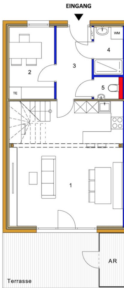
Erdgeschoss M1:75
