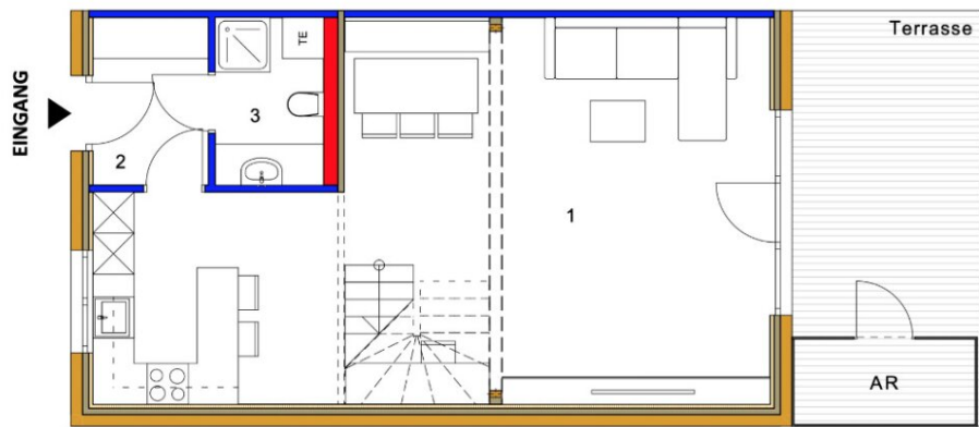
Erdgeschoss M1:75
