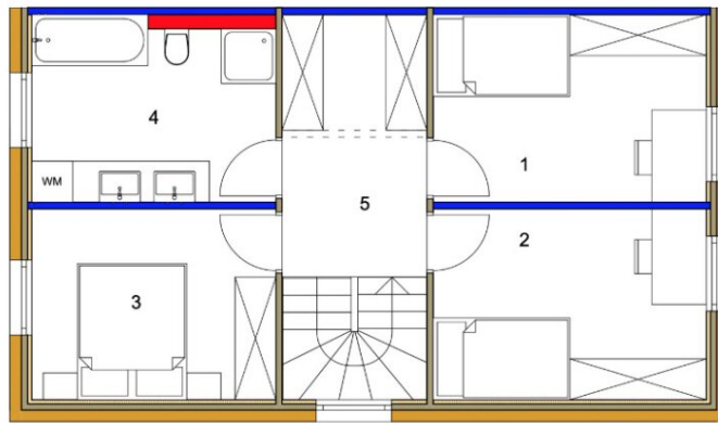
Obergeschoss M1:75
