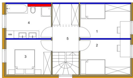
Obergeschoss M1:75
