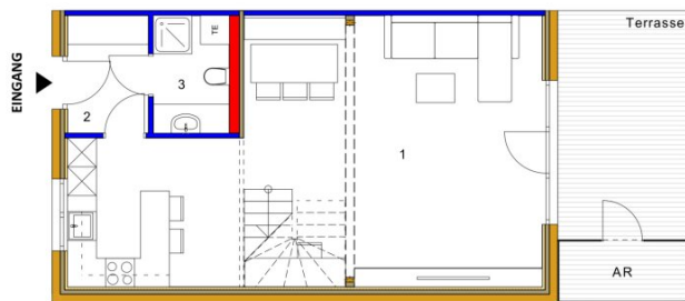
Erdgeschoss M1:75
