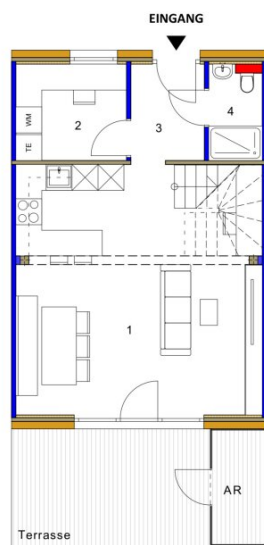
Erdgeschoss M1:75
