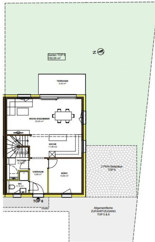
ERDGESCHOSS
