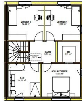
OBERGESCHOSS
