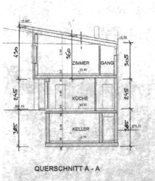
Schnitt A-A
