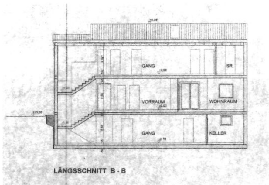
Schnitt B-B
