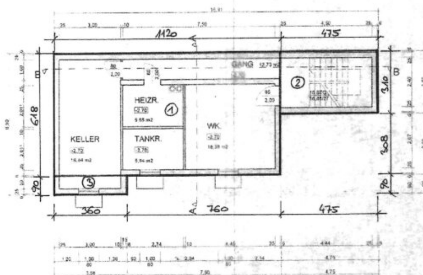
KELLERGECHOSS
