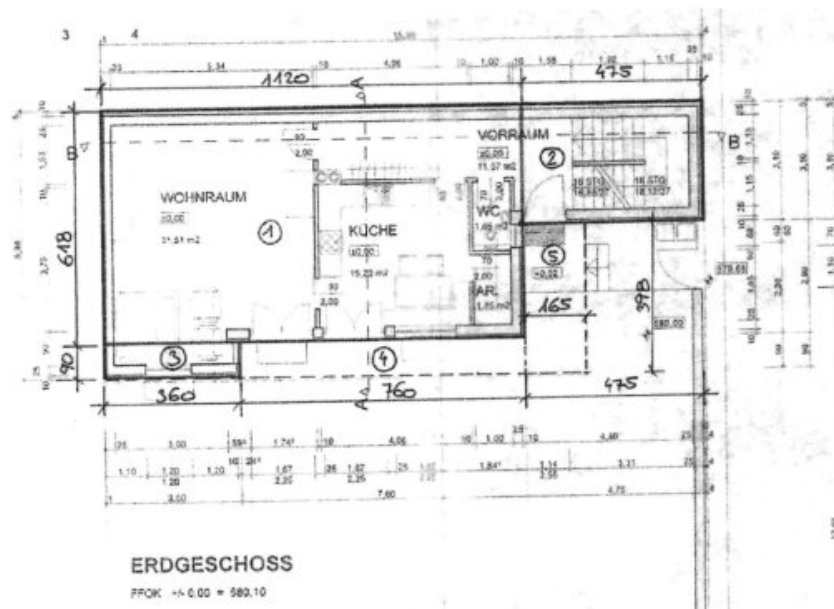
Erdgeschoß
