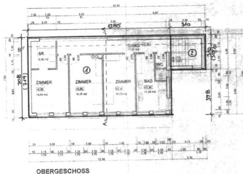
Obergeschoß
