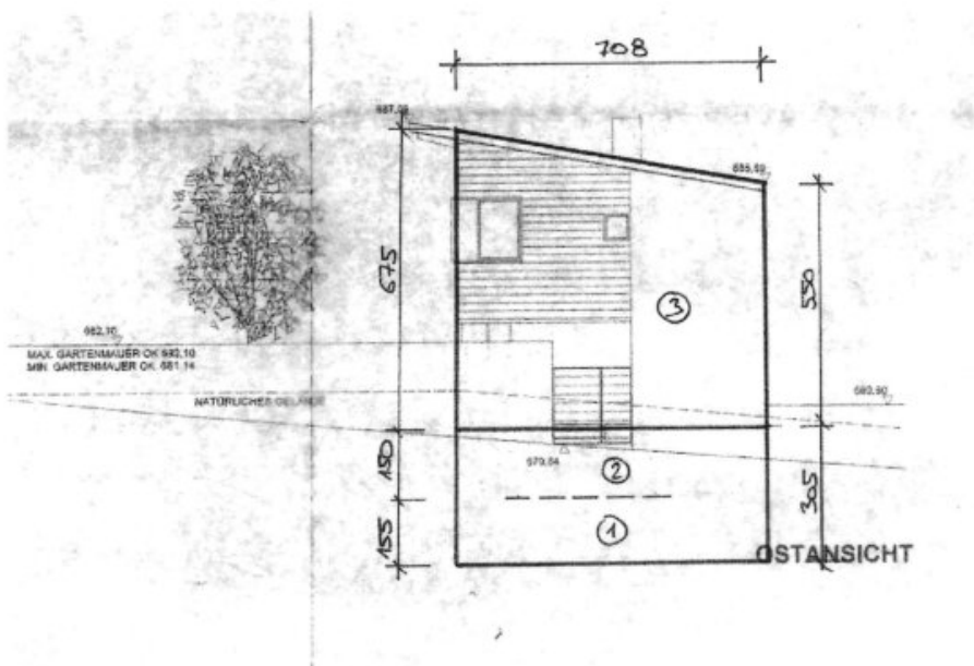
Ostansicht
