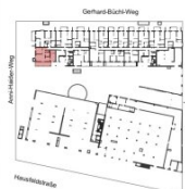
Architectural Floor Plan Details: ZIMMER 2: 11.88 m² Parkett ZIMMER 1: 11.66 m² Parkett WOHNRAUM: 19.61 m² Parkett KÜCHE: 6.56 m² Parkett BAD: 5.64 m² Fliesen WC: 2.16 m² Fliesen VORRAUM: 5.57 m² Parkett TERRASSE: 20.23 m² Ringelsteinen im Gefälle Freifläche: 68.30 m² Rasen Übersichtsskizze: Overview sketch of the building footprint.
