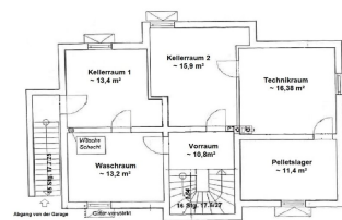
Kellergeschoss Skizze
