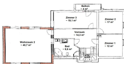
Obergeschoss-Skizze
