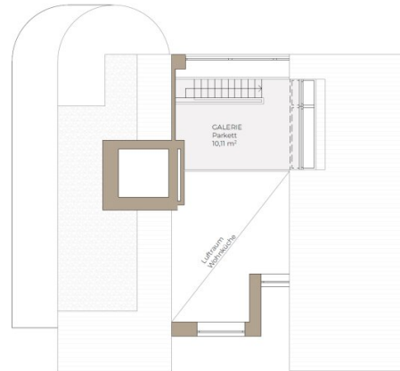
Galeriegeschoss
