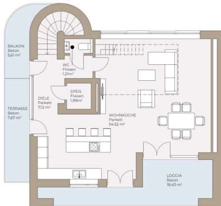
Dachgeschoss
