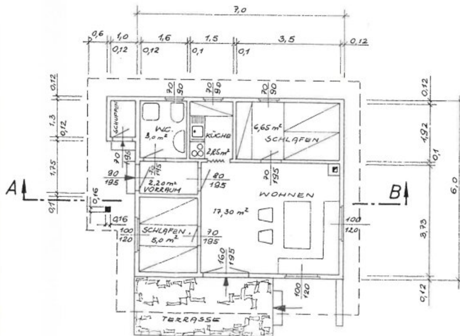
GRUNDRISS M 1:100
