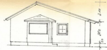
SUD-ANSIGHT
