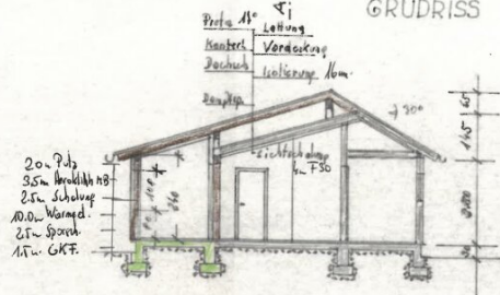
SCHNITT A:B
