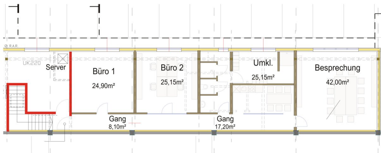
GRUNDRISS OG 1:100
