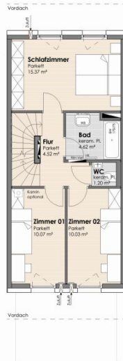
OBERGECHOSS
