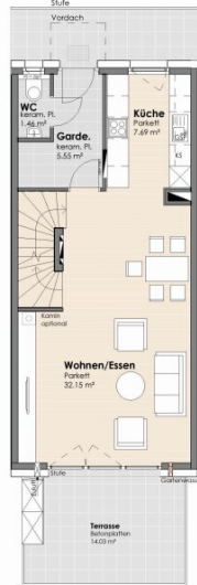
ERDGECHOSS
