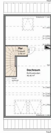
DACHGECHOSS
