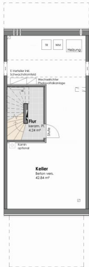
KELLERGECHOSS
