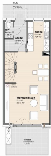
ERDGESCHOSS
