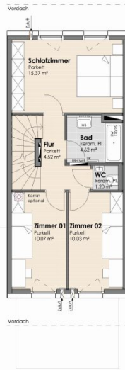
OBERSGESCHOSS
