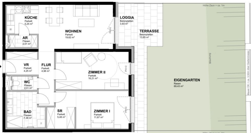
Übersichtsplan Erdgeschoss
