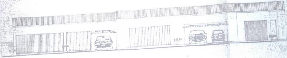
WESTANSICHT
