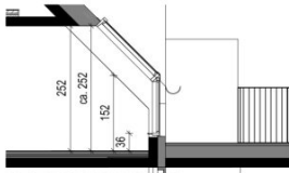
Schnitt 39 A
