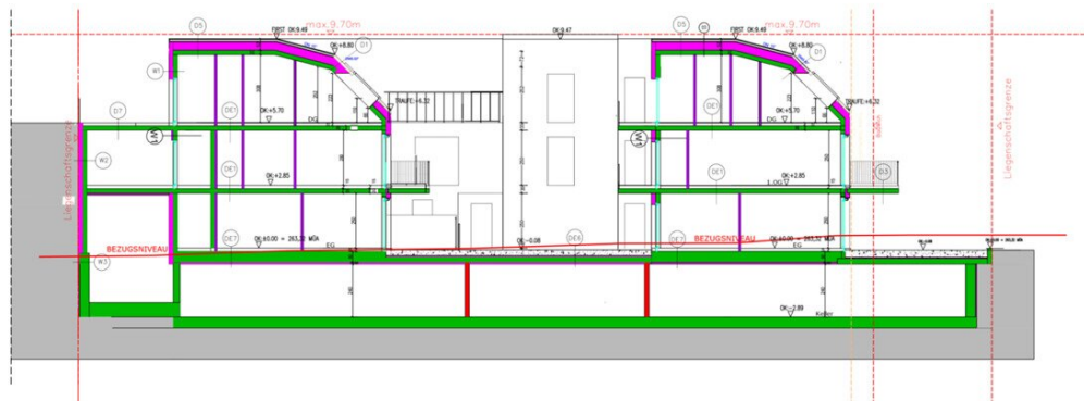
SCHNITT C-C
