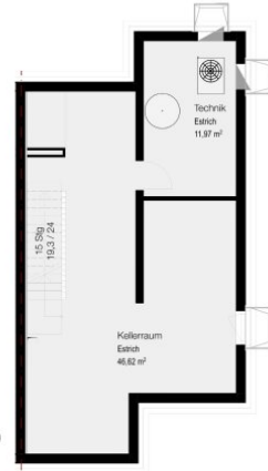
Kellergeschoss
