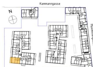
ÜBERSICHTSPLAN-1.OG
