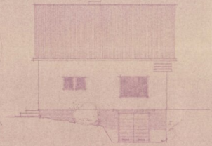
Westaufsicht
