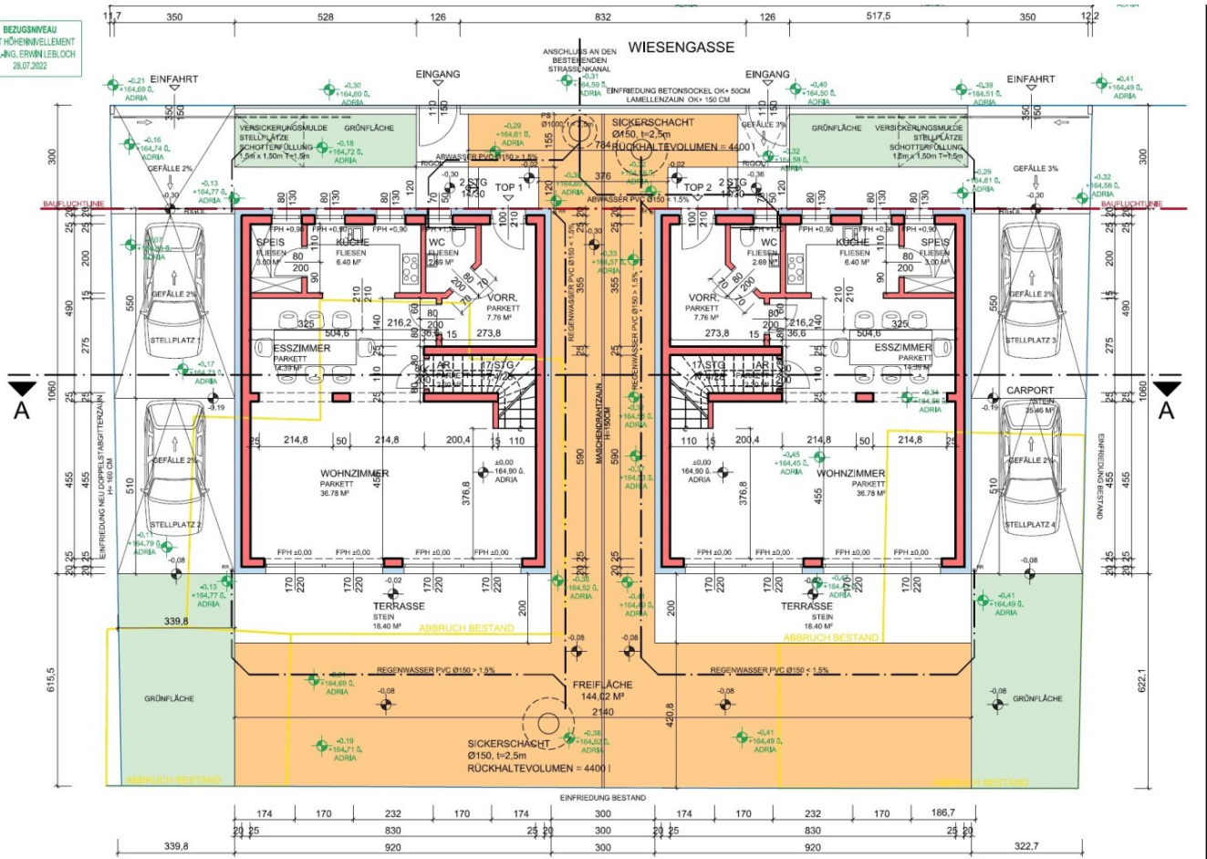
ERDGESCHOSS M 1:100
