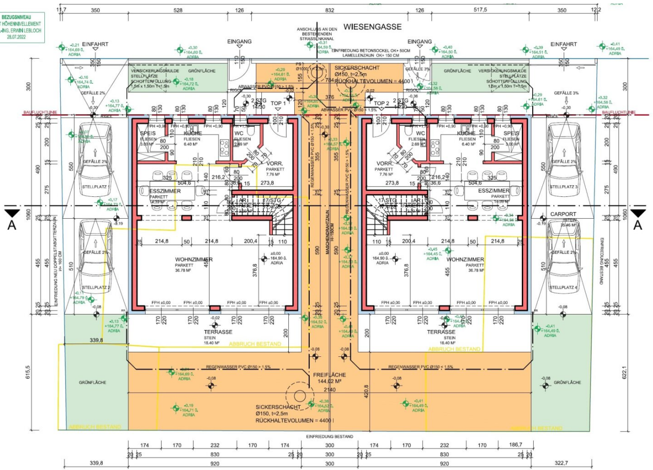
ERDGESCHOSS M 1:100
