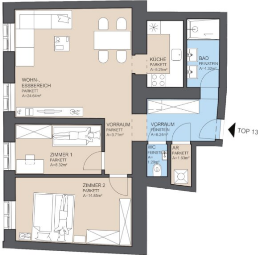
2.OBERGESCHOSS
