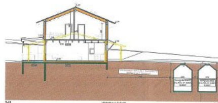
Wohnhaus Schnitt
