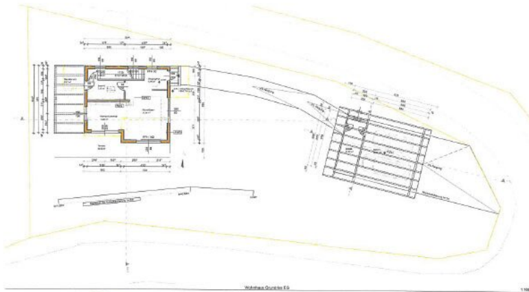
Wohnhaus Grundriss EG
