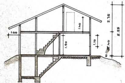
SCHNITT A-A
