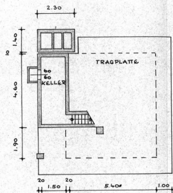
KELLERGECHOSS
