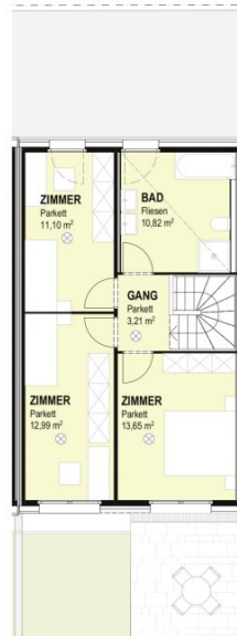
GRUNDRISS OG
