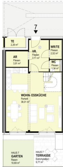
GRUNDRISS EG
