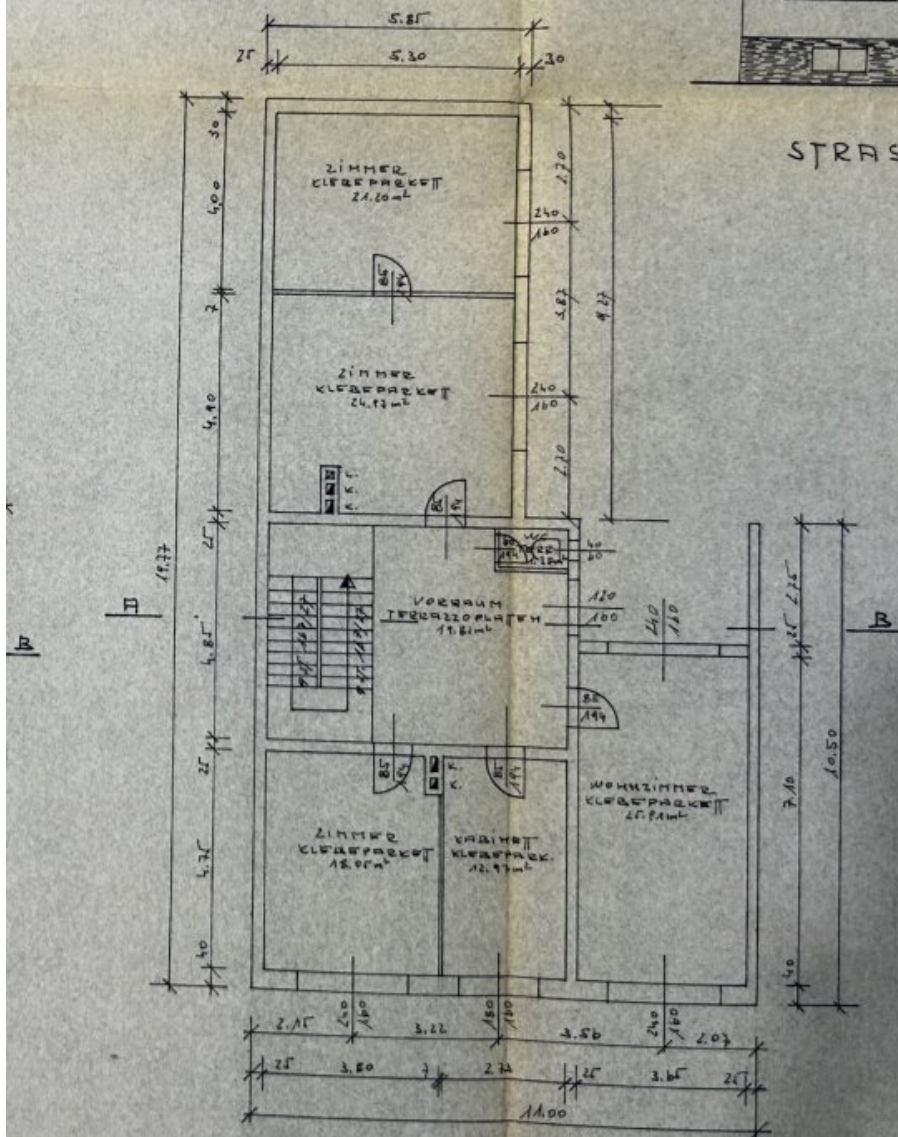
OBERGESCHOSS-GRUNDRISS
