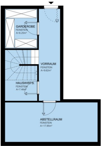
2. UNTERGESCHOSS
