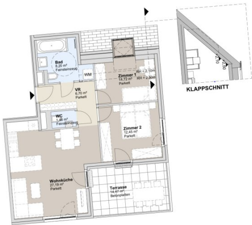
2. DACHGESCHOSS GARTENBAUKÖRPER
