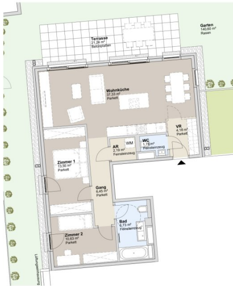
ERDGESCHOSS GARTENBAUKÖRPER
