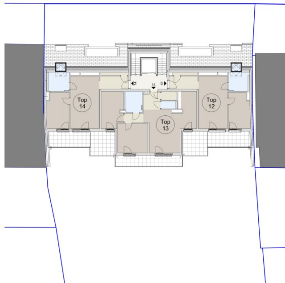
3. OBERGESCHOSS 1 : 200
