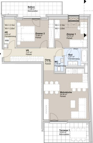
1. DACHGESCHOSS STRASSENBAUKÖRPER
