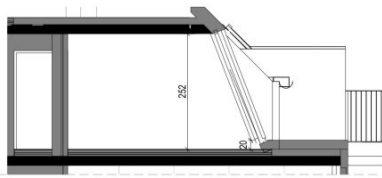
Schnitt 41.B
