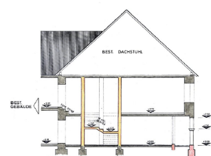
SCHNITT
