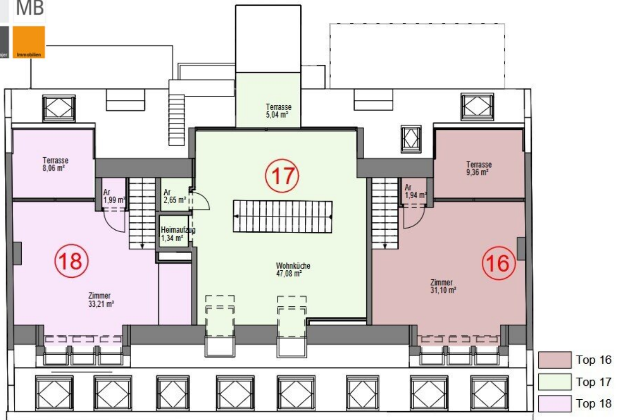
2. DACHGESCHOSS M 1 : 125
