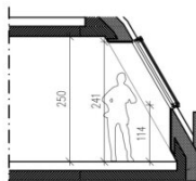
SNITT B3
