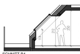
SCHNITT B4
